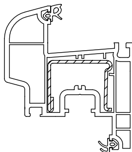
Уплотнитель притвора
