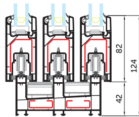
Стулка SL 39/82 098
