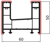
Рама SL 60/50 094
