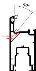
Стулка SL 39/82 098
