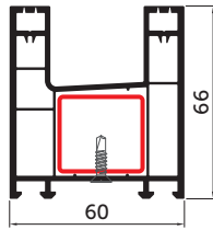
Рама SL 60/66 095
