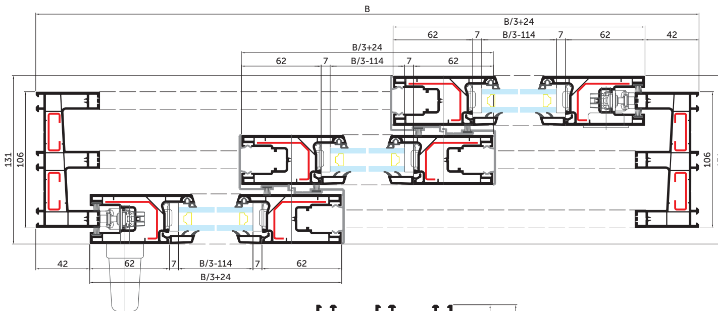
Схема 5 3 стулки зсувні
