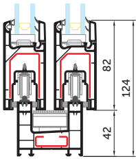
Рама SL 60/50 094
