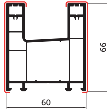
Рама SL 60/66 095
