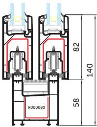
Рама SL 60/66 095
