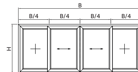
Схема 2 2 стулки зсувні, 2 стулки фіксовані
