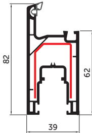
Стулка SL 39/90 099
