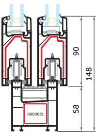
Рама SL 60/66 095
