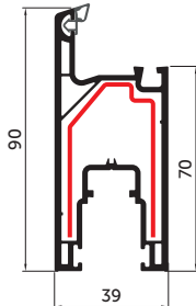
Стулка SL 39/90 099
