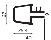
З'єднувач-підсилювач
