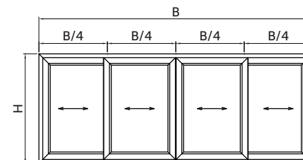
Схема 4 4 стулки зсувні
