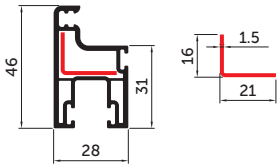
Стулка москітної сітки
