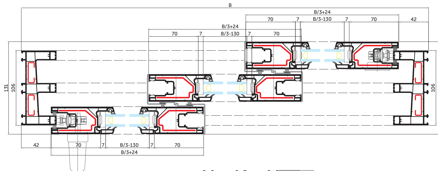
Схема 5 3 стулки зсувні
