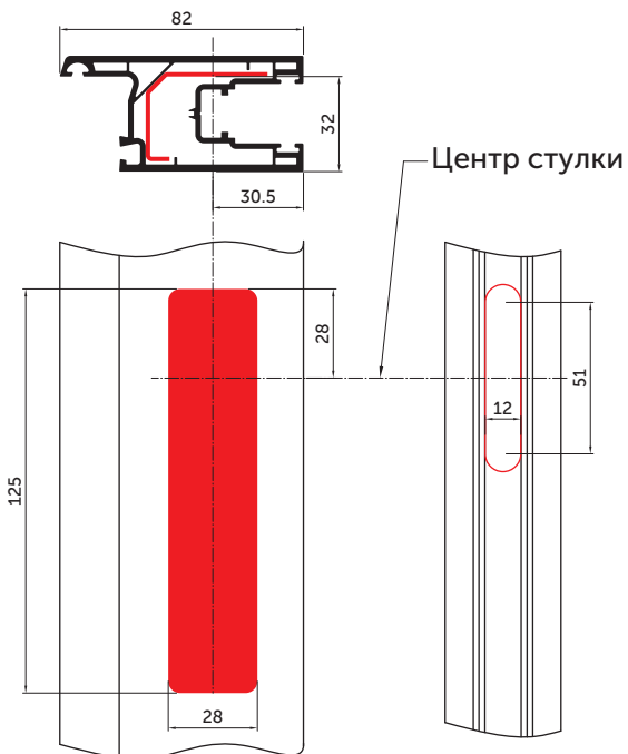
Отвори під дорнмасс 7.5 мм
