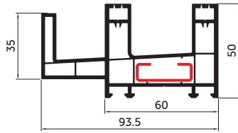
Рама SL 106/50 096
