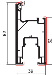
Стулка SL 39/82 098
