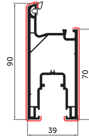
Стулка SL 39/90 099
