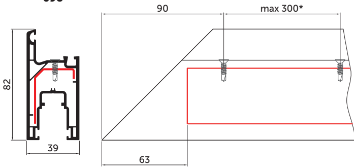
Стулка SL 39/82 098
