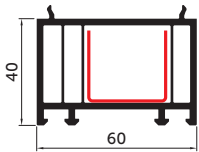
Розширювач рами
