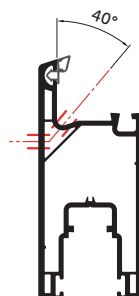
Стулка SL 39/90 099
