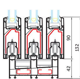
Рама SL 106/50 096
