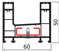
Рама SL 60/50 094
