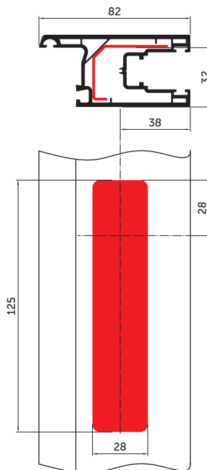
Отвори під дорнмасс 15 мм
