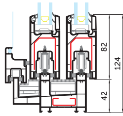
Рама SL 60/50 2+1 100
