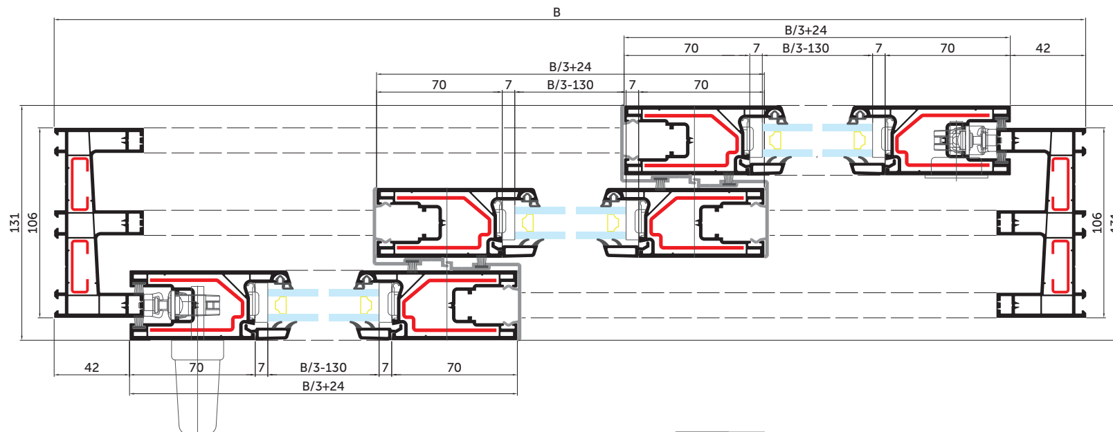
Схема 5 3 стулки зсувні
