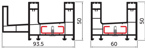
Рама SL 60/50 2+1 100
