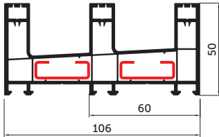
Рама SL 60/66 095
