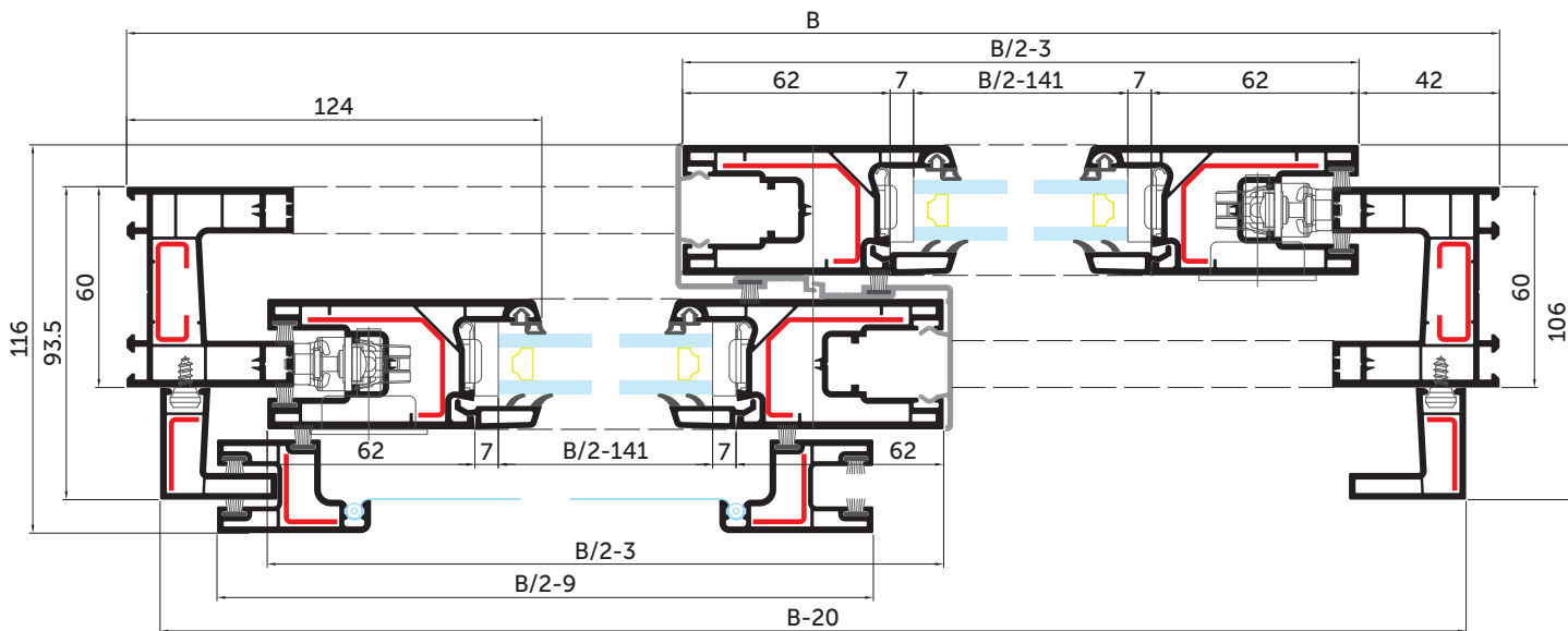
Схема 3 2 стулки зсувні
