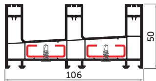
Рама SL 106/50 096
