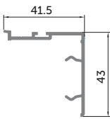
Заглушка стулки SL алюмінієва Біла RAL9016 D000191 Коричнева RAL8017 D000192 Антрацит RAL7016 D000193
