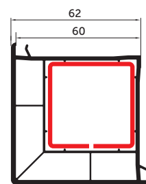
Кутовий з'єднувач
