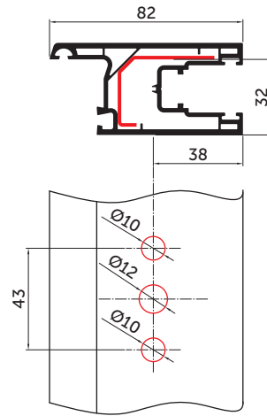
Отвори під дорнмасс 15 мм
