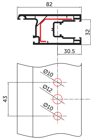
Отвори під дорнмасс 7.5 мм
