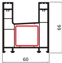
Стулка SL 39/82 098
