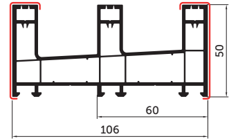
Рама SL 106/50 096
